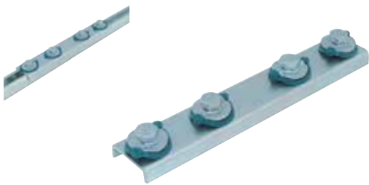
Walraven RapidRail® Schienenverbinder (ev)
