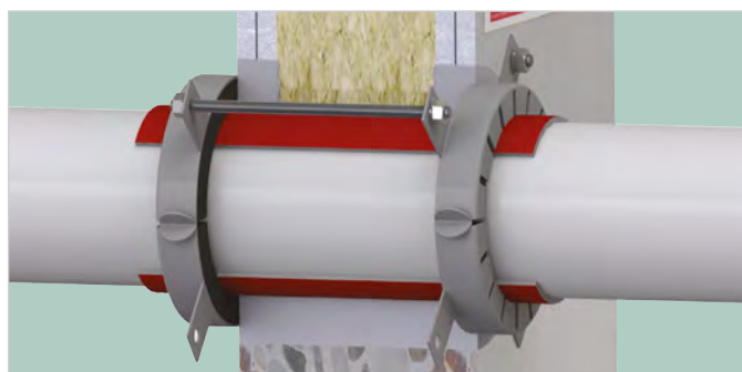
Anwendung in Massivwänden und -decken.
