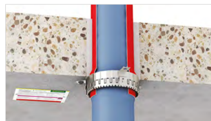
schallgedämmte Abwasserrohre mit PE-Schallschutzschlauch
