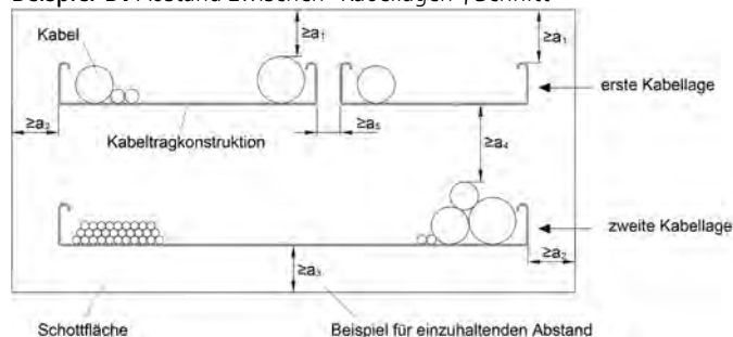
Beispiel D: Abstand zwischen "Kabellagen"; Schnitt
