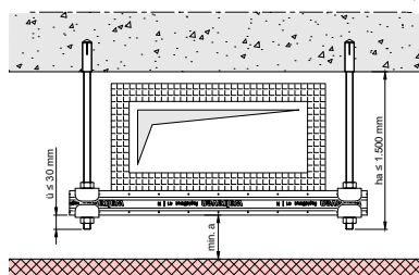
Schienenfuß und Profilschiene
