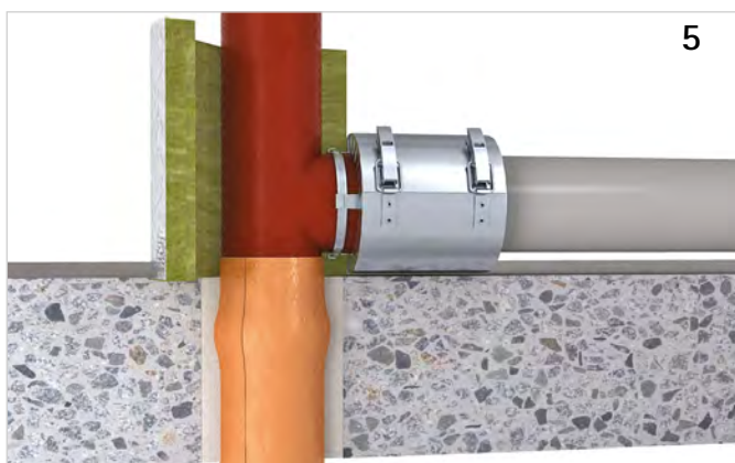
Walraven Pacifyre® Isoliermatte ( H \geq 250 \text{ mm} ) um das Rohr legen und mit Aluband sowie Bindedraht verschließen.
