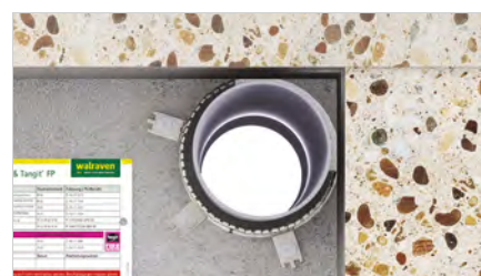
Besonders geeignet für Ecklösungen - 2/3 Umwicklung (abhängig von Rohrgruppe gemäß Verwendbarkeitsnachweis)
