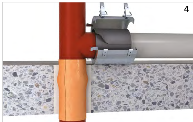
Blechgehäuse der Walraven Pacifyre® KonFix Hülse öffnen, bündig um das Band legen, Laschen schließen und mit dem Metallspannband fest am Rohr fixieren.
