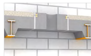
Stahlträgerverbunddecke
