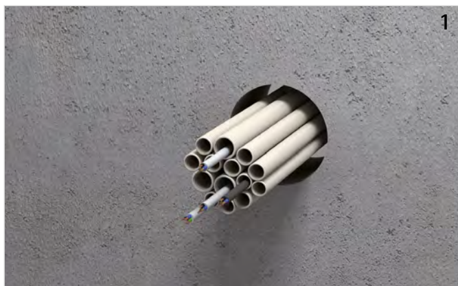
1 Kabelleerrohre durch das Bauteil führen und außerhalb des Bauteils mit Kabelbinder o. ä. bündeln.
