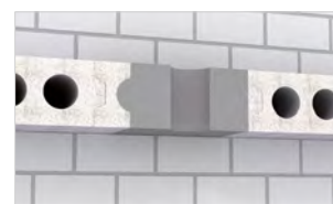
Porenbetondecke (ggf. mit Hohlkammern)
