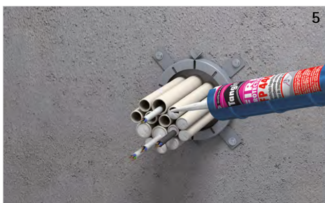
5 Die unbelegten Leerrohre und andere Restöffnungen rauchgasdicht mit z. B. Walraven Pacifyre® Sibralit DX Brandschutz-Fugenfüllmasse verschließen.
