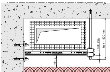
Wandkonsole mit Luftkanal oder Kabeltrasse
