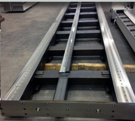
Fahrbahnrahmen 4 to.
