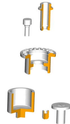
Fließpressteile
