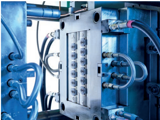
Heißkanal-Spritzwerkzeug mit 12 Kavitäten, mit 500.000 Schuß garantierter Ausbringung
