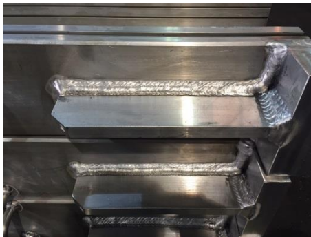
Aluminium-Schweißbaugruppe
