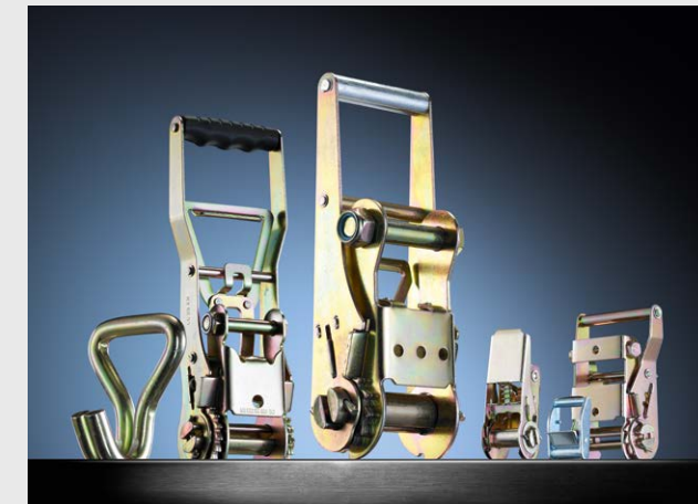
Spannelemente zur Ladungssicherung Load restraint assemblies
