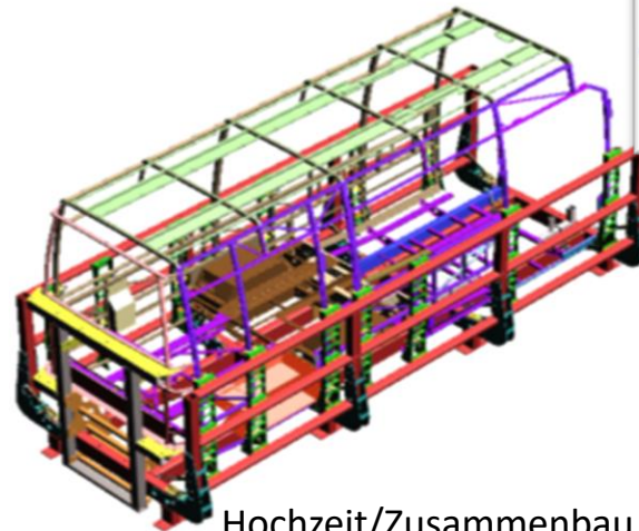
Hochzeit/Zusammenbau
