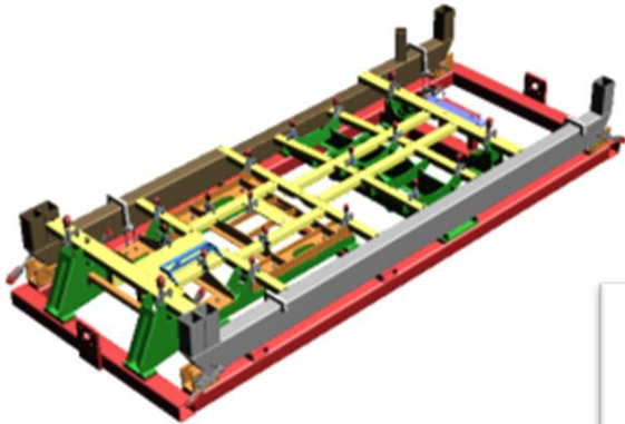
Unterbau/Chassis
