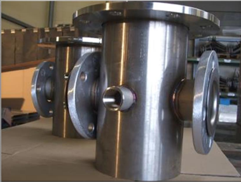
WIG-Naht Edelstahl
