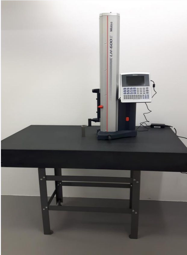
Mitutoyo Linearer Höhenmesser LH-600E
