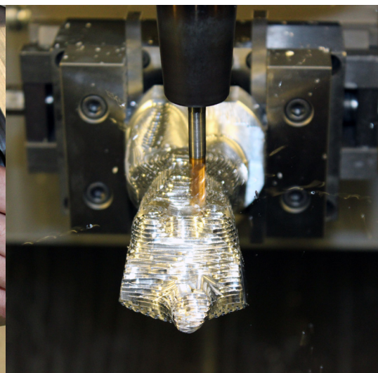
Umformwerkzeuge
