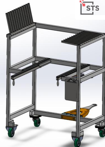
Kommissionierwagen Unterbodenblech
