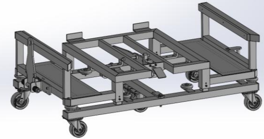
Transportwagen FTS-geführt
