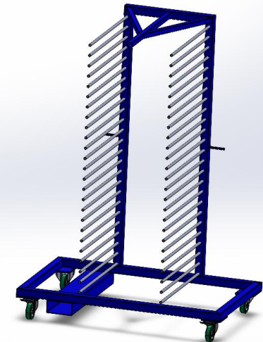
Kommissionierwagen Seitenscheiben
