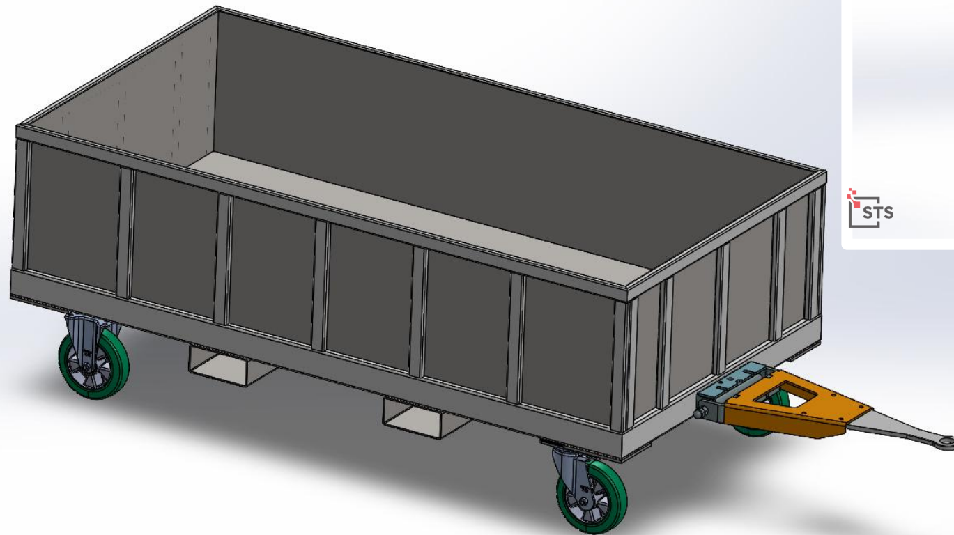
STS Transportwagen
