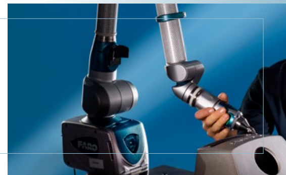
Messarm Modell FARO ARM EDGE 2.7 für dreidimensionale Messungen mit Scanning-, Analyse- und Reporting-Software PolyWorksInspector
