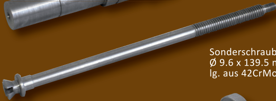
Führungsbolzen Ø 25 x 72 mm lg. aus 115CrV3
