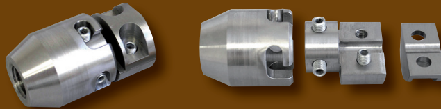
Stellschraube 3h7 x 94 mm lg. SW 4.2 (aussen) sowie SW 2 Innensechskant
