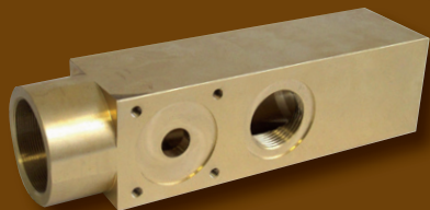
Gehäuse 65 x 65 x 250 mm aus CuZn39Pb3
