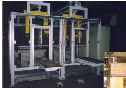
Handhabungsanlage zum Tauchen von Zylinderkopf-Kernen
