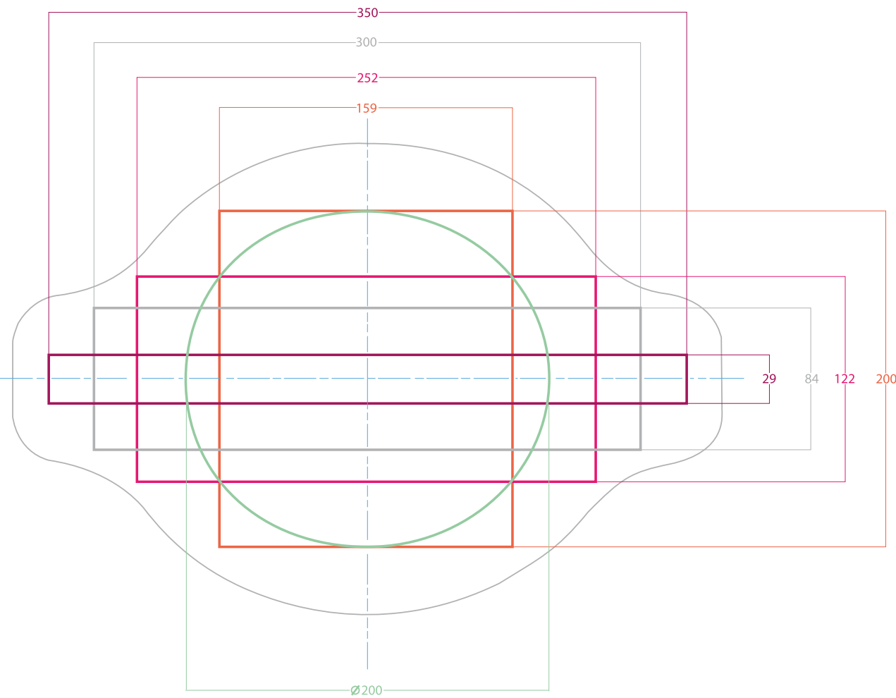
Verfügbare Querschnittsgrößen.
