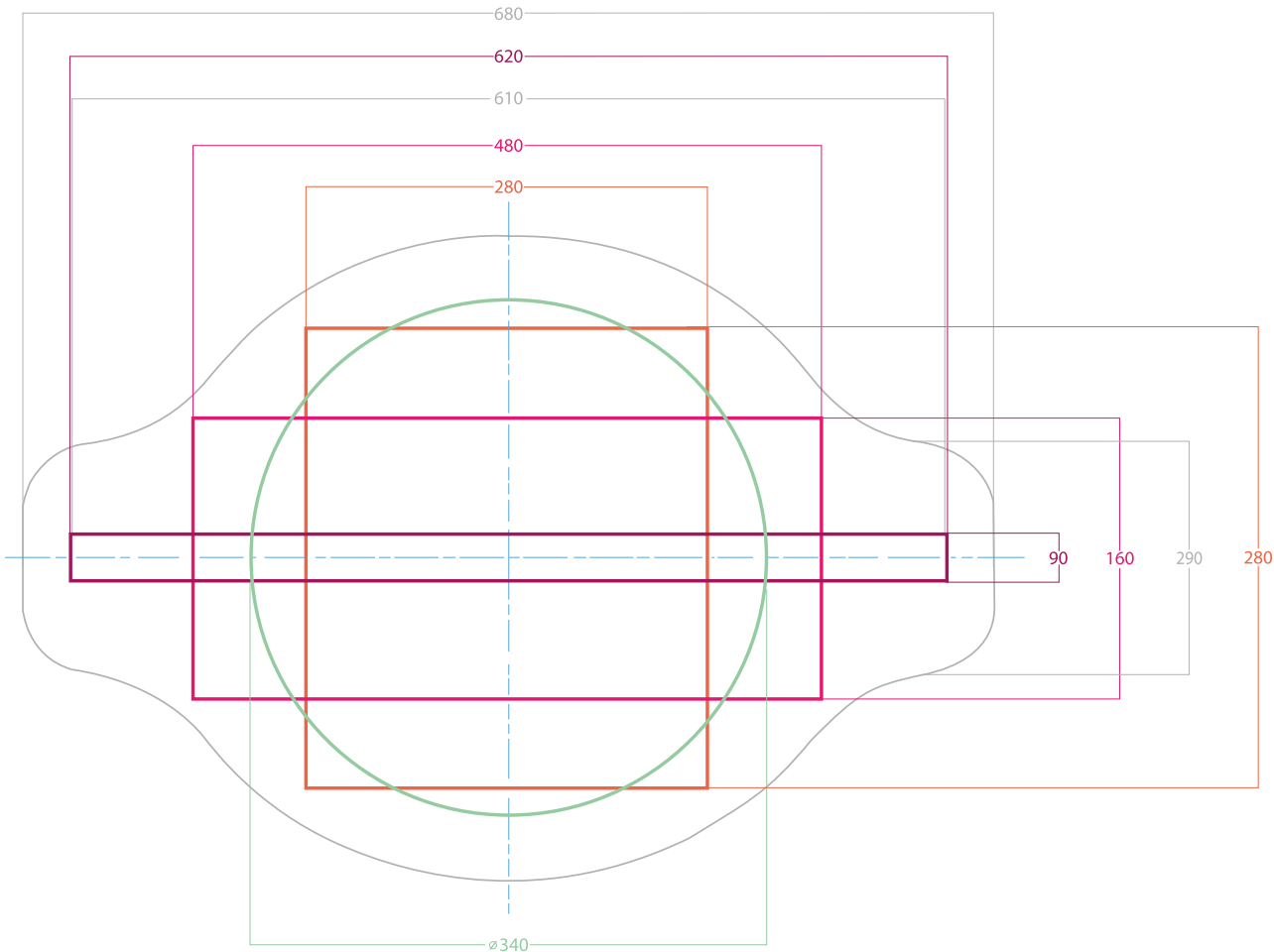
Verfügbare Querschnittsgrößen.
