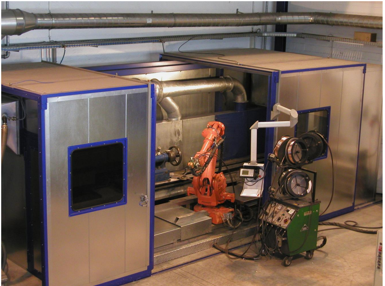
Schallschutzkabine für thermische Beschichtungen mit 7 Achsen Roboter
