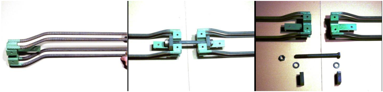
Spannelemente für Rechteck- / Rundbehälter aus Beton - einzeln oder im Set beziehbar
