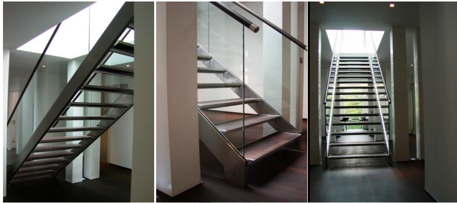
Raumspartreppe in einem Geschäftshaus
