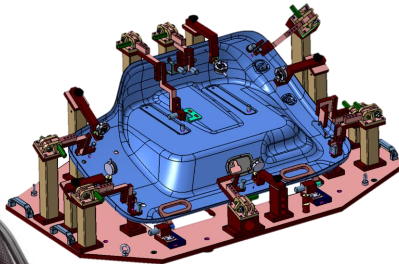
Tiefziehen - Abdeckhaube
