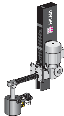
Schnellspannsysteme mit Schubkette
