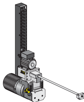
Winkelspanner mit Spindeltrieb
