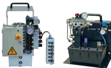
Baureihe 5 2.5 l/min., 400 bar
