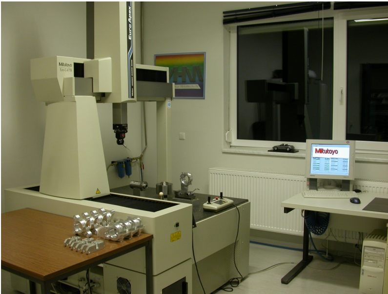
CNC - Koordinatenmessgerät Messbereich X705, Y705, Z605
