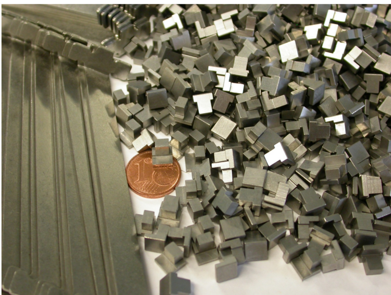
Fixierelemente für Turbolader
