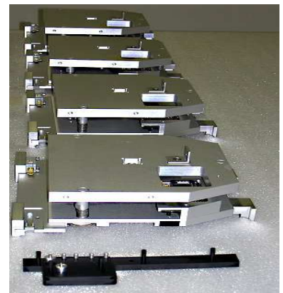
Montagebeispiel einer Baugruppe
