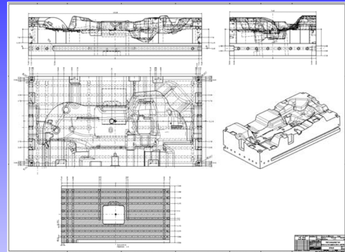
Fertigungszeichnungen
